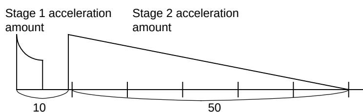
Fig. 4.6.5 (d) Stage 2 end scale factor
