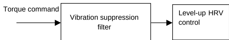
Fig. 3.4.1 (d) Vibration suppression filter
