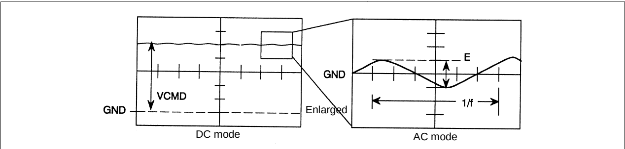
Fig. 4.19 (d) Waveform of the VCMD signal
