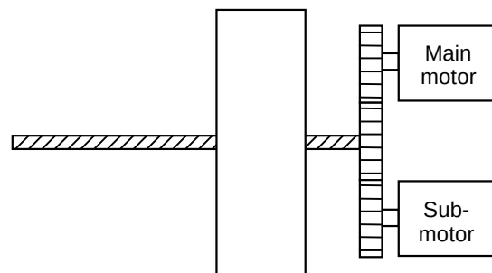
Fig. 4.17.10 (d) Example of tandem control (rigid machine system)
